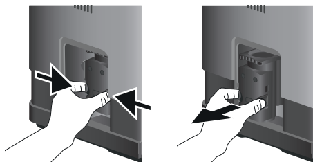
Abb. 8: Brühereinheit ausbauen
