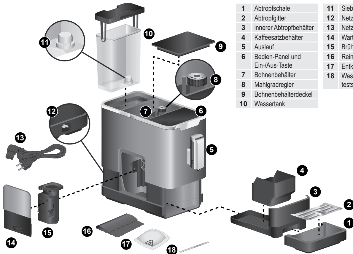
Abb. 1: Teile des Geräts
